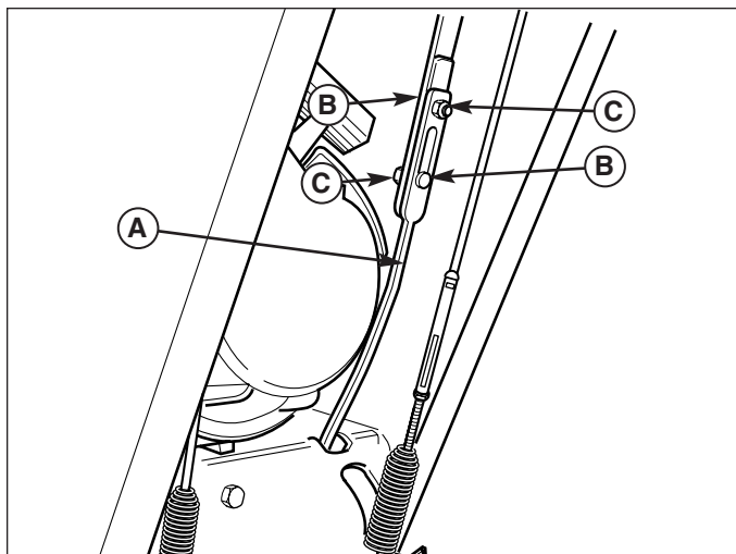
Figur 18. Hastighetsväljare och länksystemet för skruvens drivmekanism
